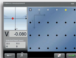
Programa de planitud. Medición.
