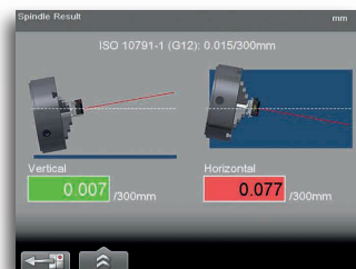
Programa de husillo. Resultado.
