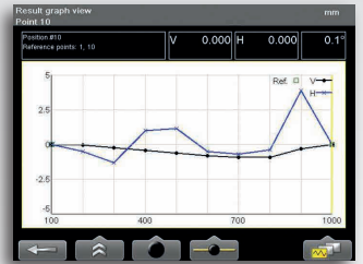
Programa de rectilineidad. Gráfica de resultados.
