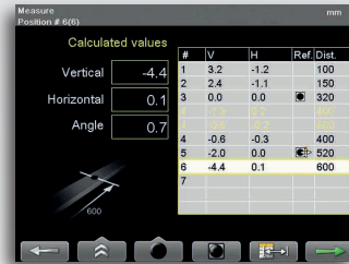
Programa de rectilineidad. Medición.
