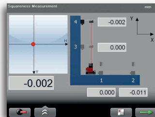
Programa de perpendicularidad. Medición.
